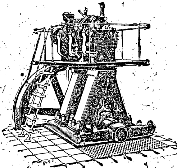
MOTOR OTTO-DIESEL
