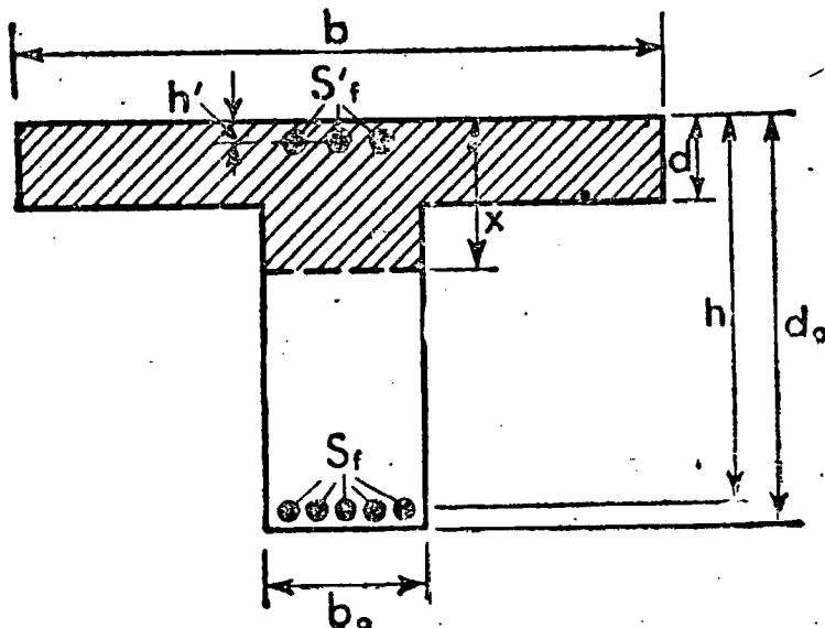
Viga T
