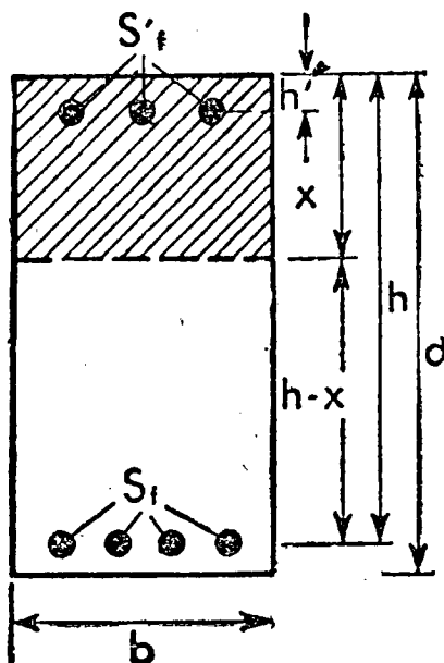
Viga de seção retangular
