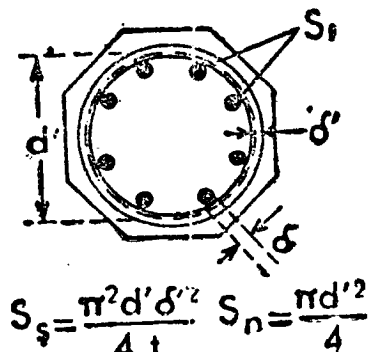
Pilar cintado
