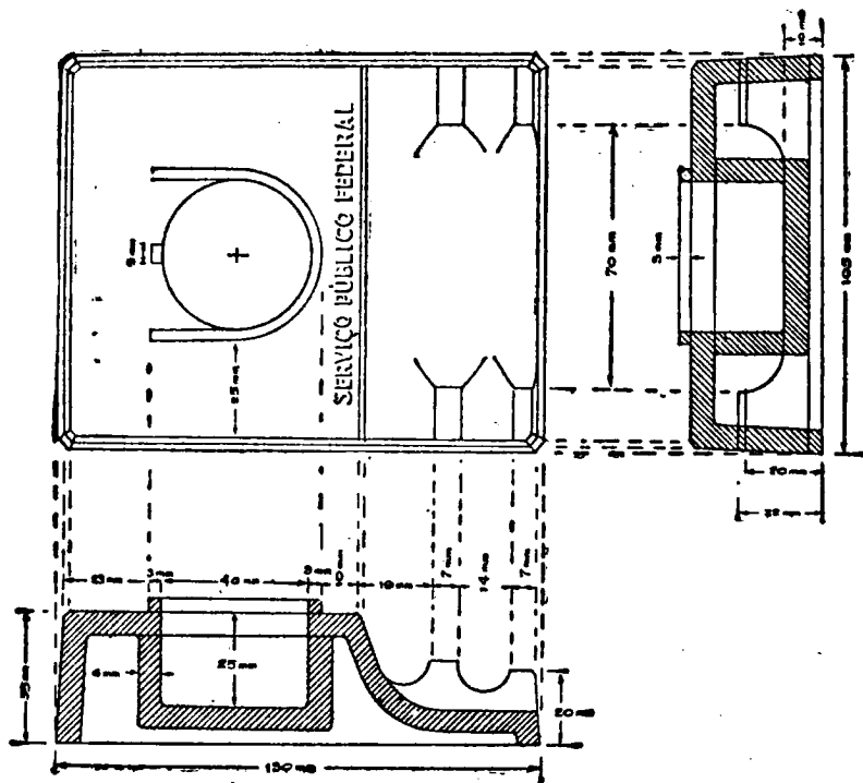
TN-1 - TINTEIRO SINGELO 105 mm x 130 mm
