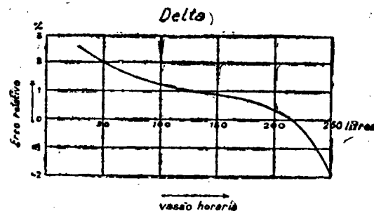
Curva característica:
